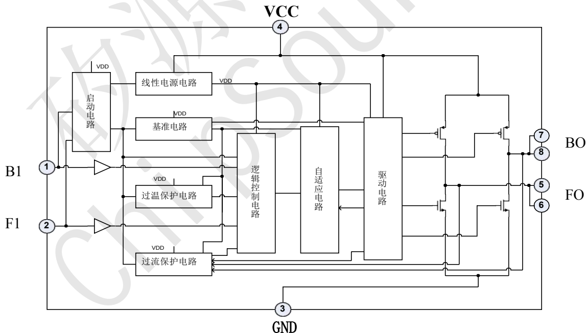
D6289框图
