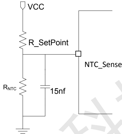
图 7 NTC 应用
