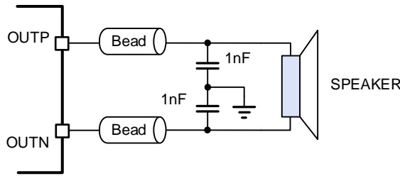
Fig.7 差分磁珠滤波输出
