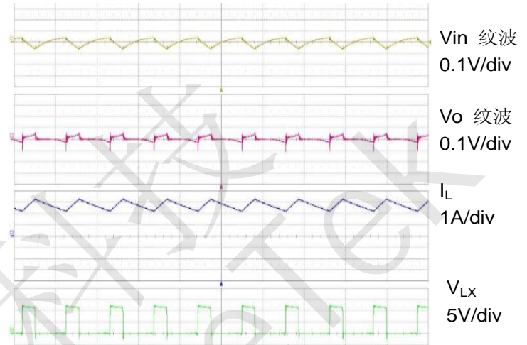
Fig.5 满载工作 2µs/div
