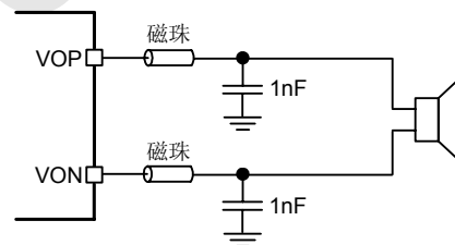
图 9 磁珠与电容
