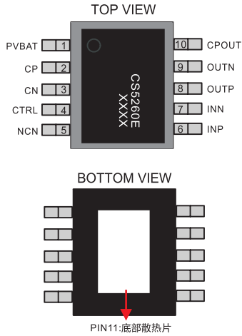
CS5260E(ESOP10 PACKAGE)
