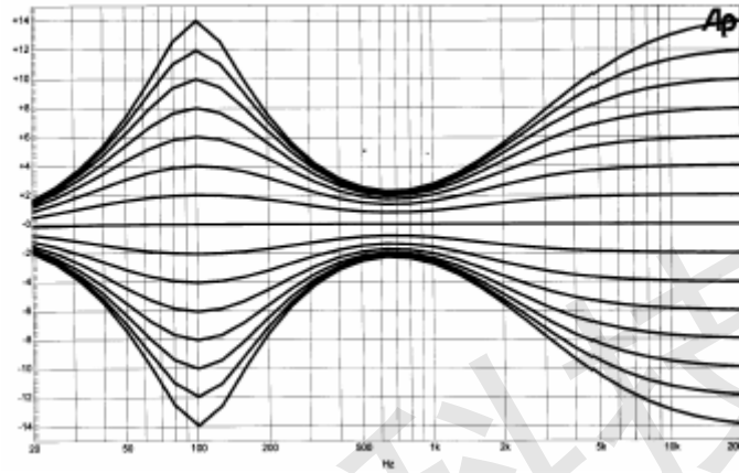
CST2314的音质频率响应图
