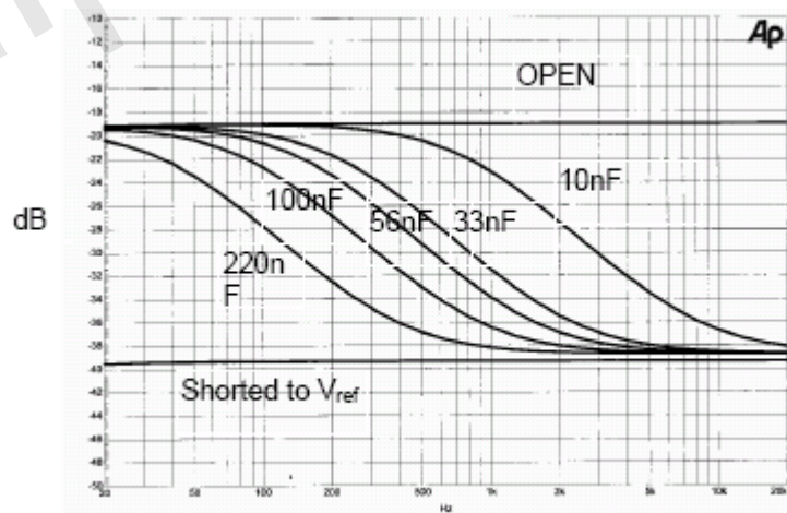
CST2314 C12、C13对响度的频率响应图 (Volume=-40Db, All other control flat)
