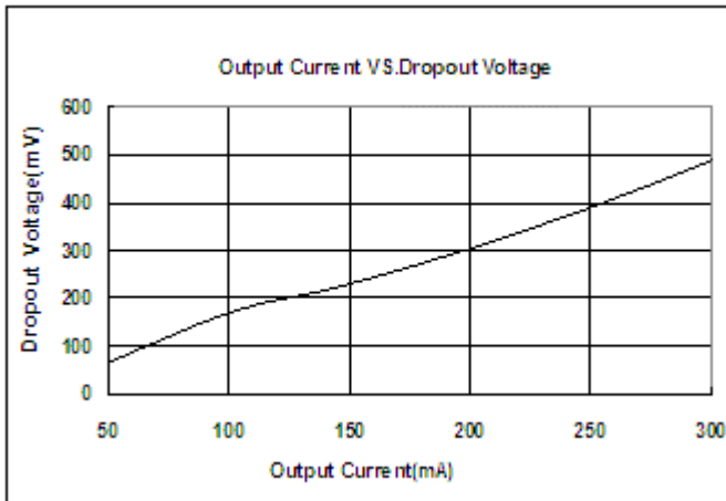
ME6219C28M5G
